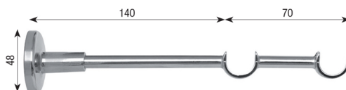
Mensola doppia aperta Ø20 Art. MS20MD/A
